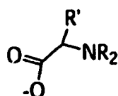
aminoacids
